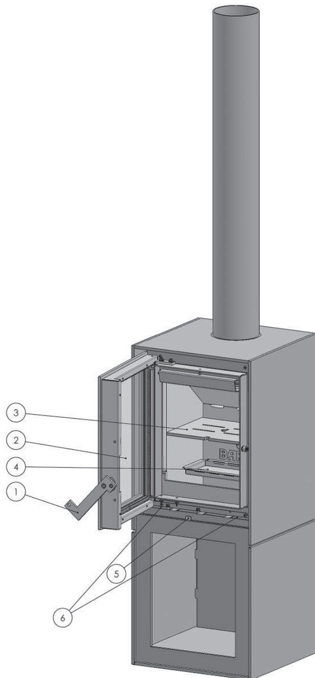
Abbildung 2: Bedienung Box mit Holzfach-Modul
