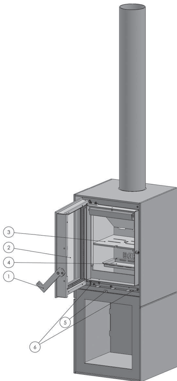
Figure 2: Commande Box avec module stockage de bûches
