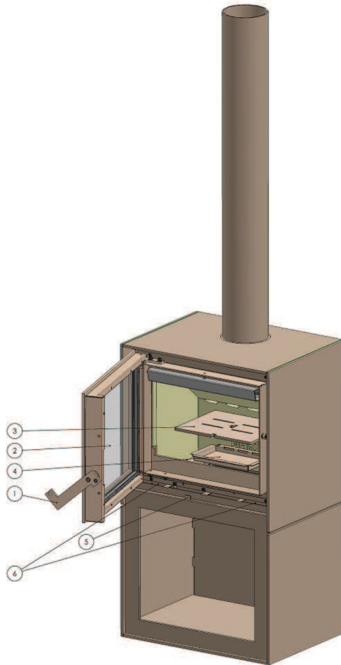
Abbildung 2: Bedienung Box mit Holzfach-Modul
