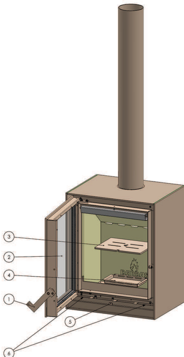
Abbildung 1: Bedienung Box
