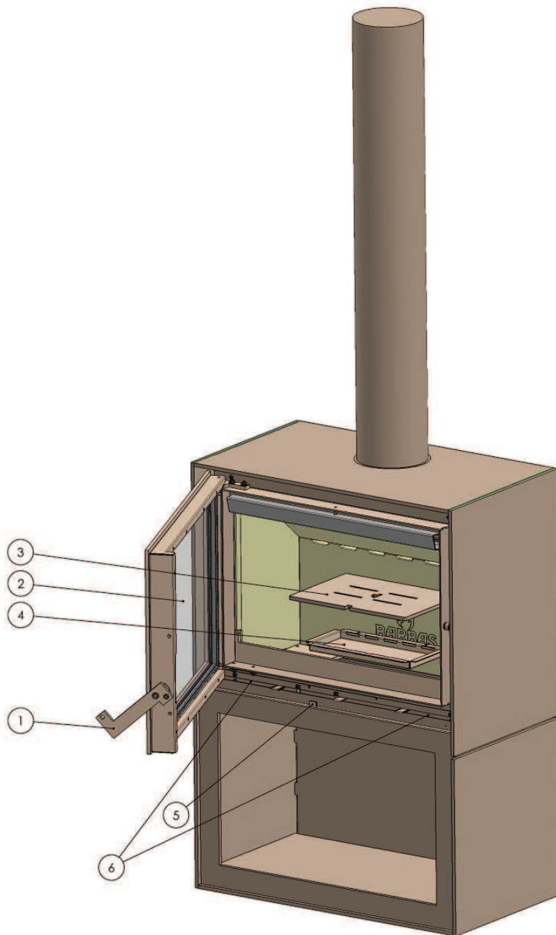
Abbildung 2: Bedienung Box mit Holzfach-Modul
