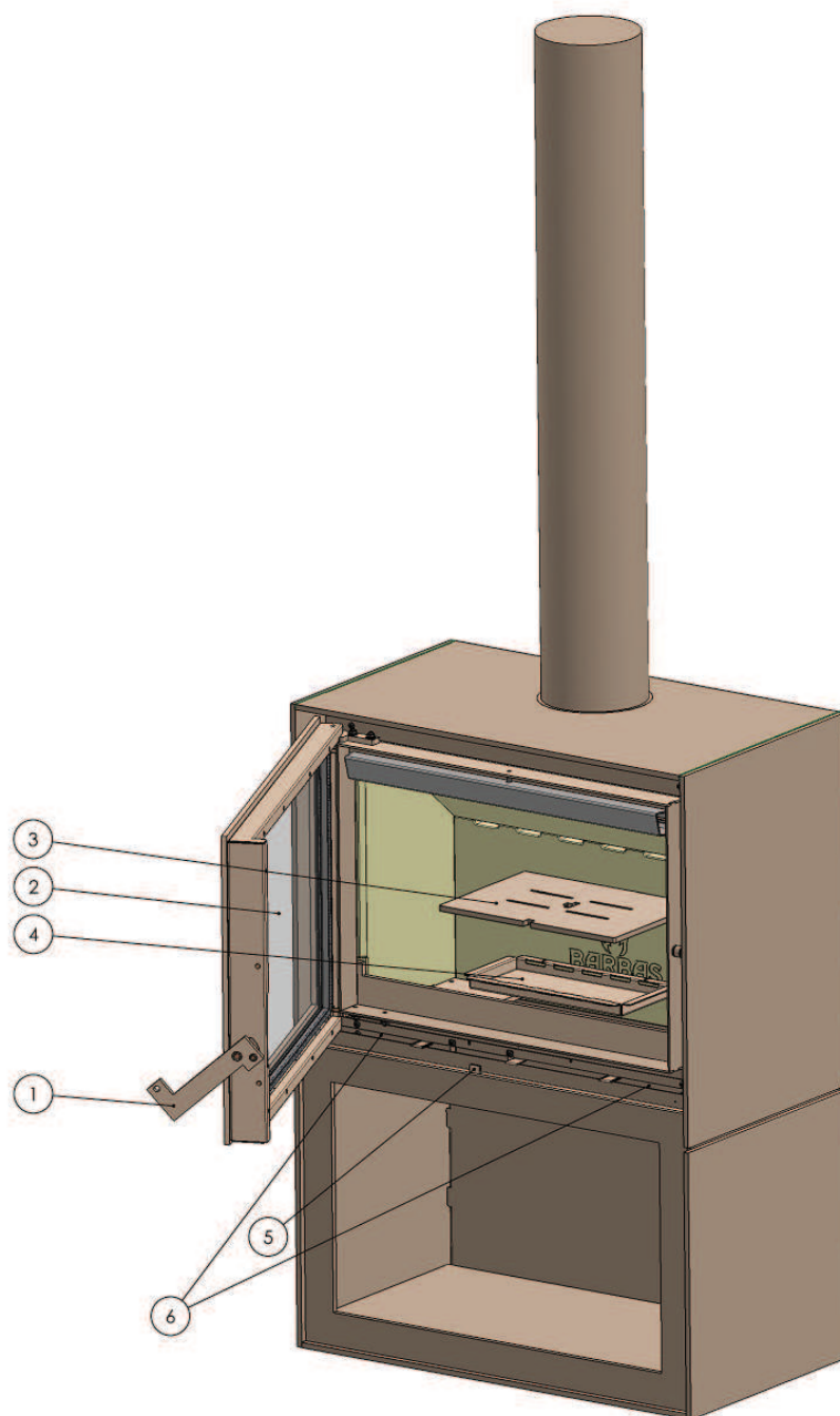
Figure 2: Commande Box avec module stockage de bûches
