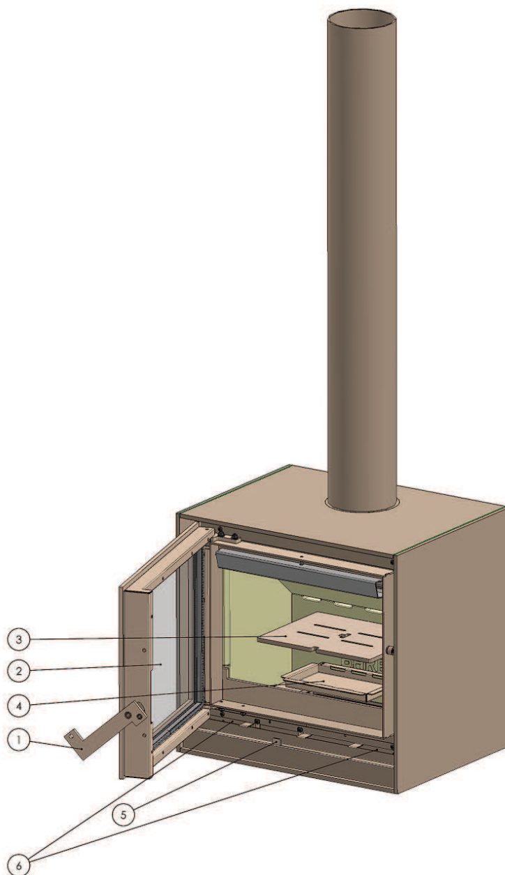
Abbildung 1: Bedienung Box
