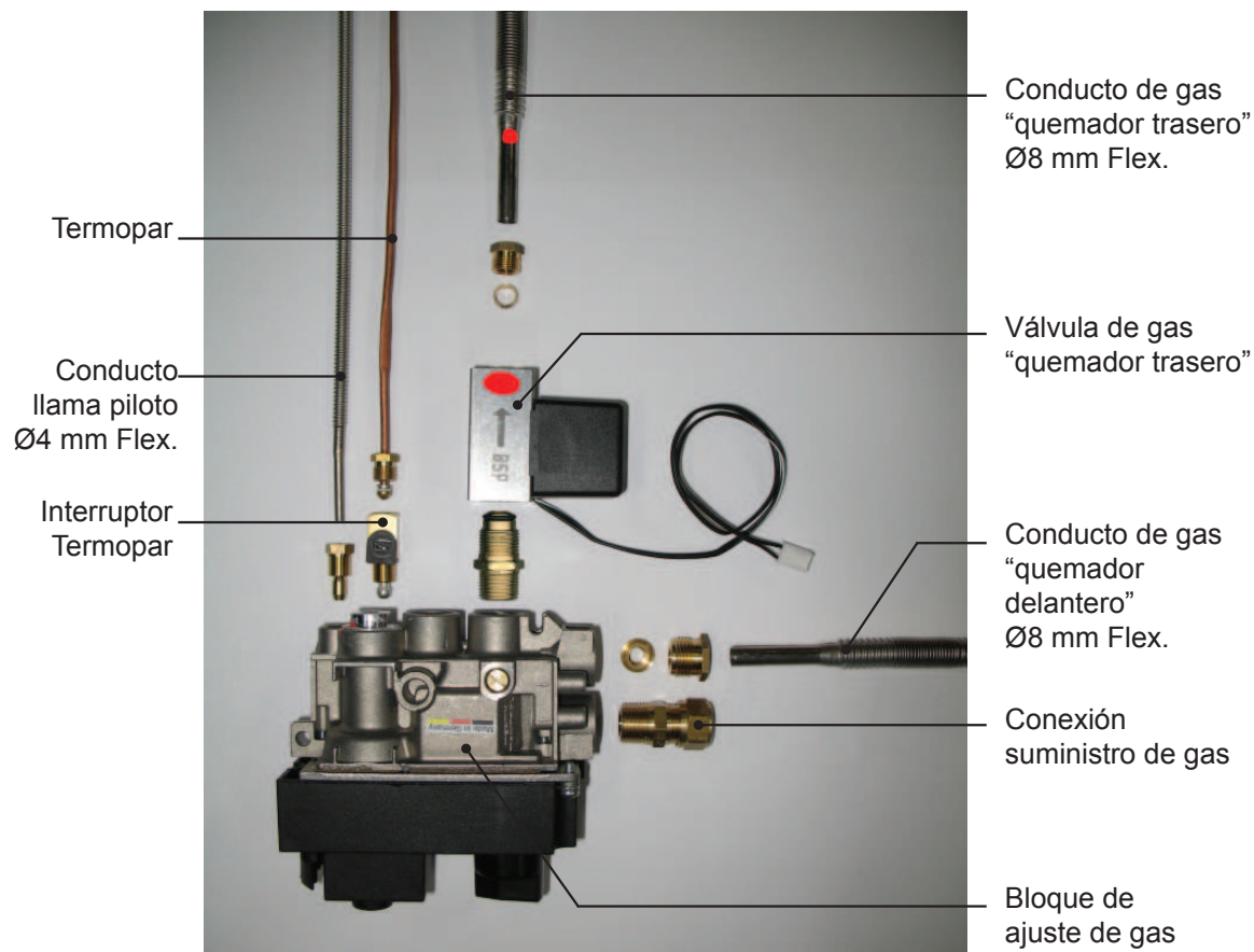
Figura 19: Bloque de ajuste de gas y válvula de gas: Conexiones de gas y el termopar
