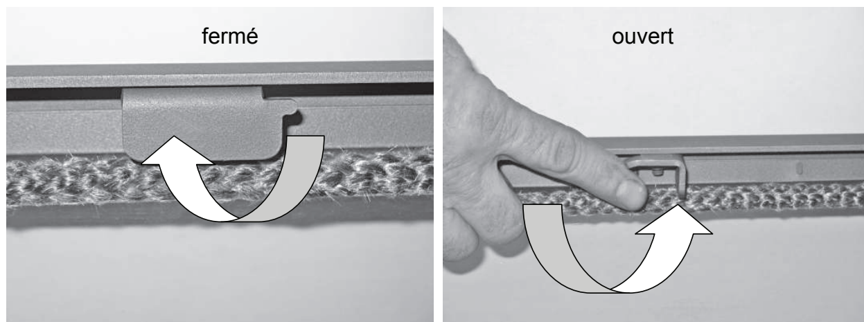
Verrouillage fermé (tourné vers la gauche) Verrouillage ouvert (tourné vers la droite)
