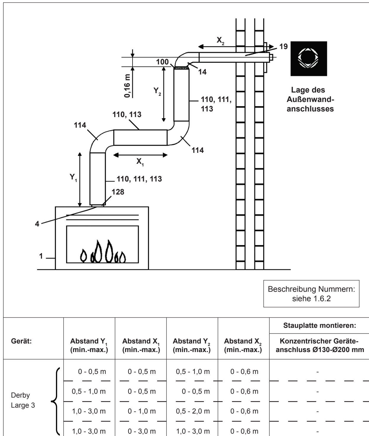
Abbildung 14: Horizontaler Außenwandanschluß
