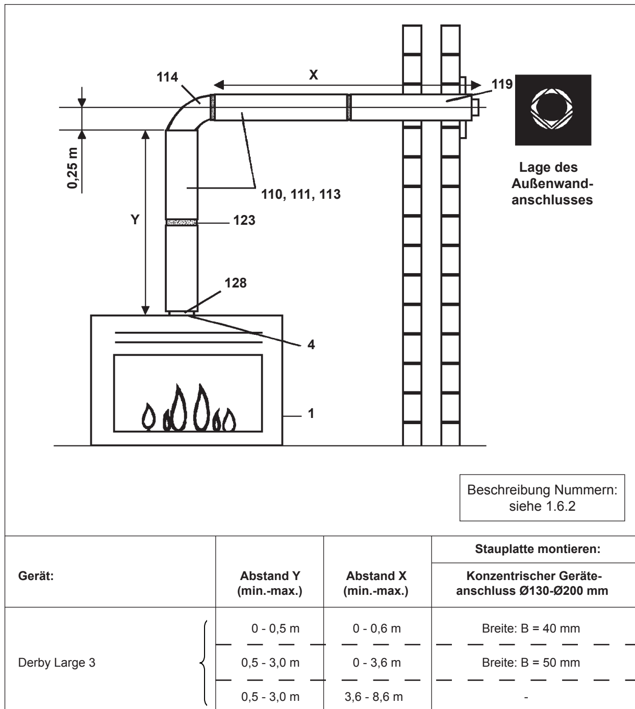
Abbildung 15: Horizontaler Außenwandanschluß
