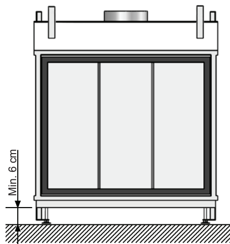
Abbildung 16: Minimal 6 cm Spiel zwischen die Unterseite des Geräts und dem Boden
