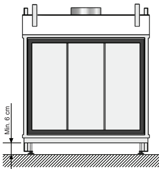
Figura 15: Mínimo 6 cm entre el suelo y la base del aparato
