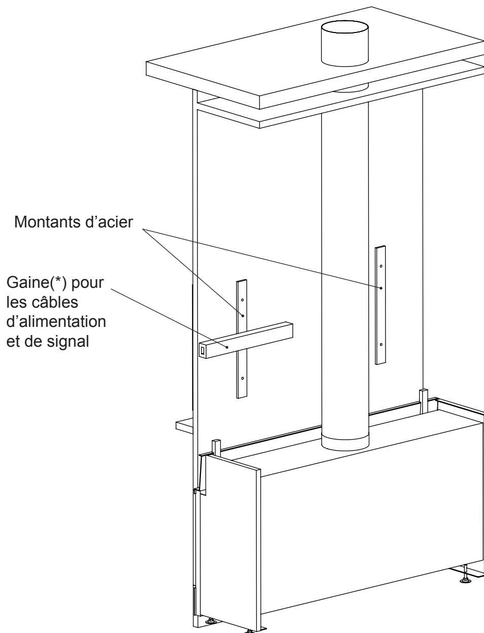
Figure 10: Installation de téléviseur au-dessus de la tablette de foyer (Foyer plat) (Installation en surface) Vue arrière
