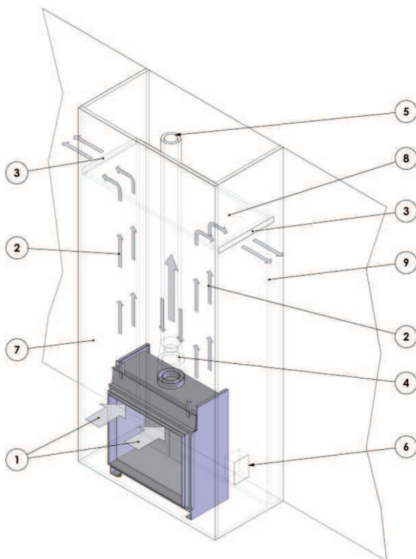
Figure 20: Appareil installé dans le manteau d'une cheminée ventilée/Enchassement Terminaison verticale d'évacuation de la fumée / source d'air de combustion au travers du toit.
