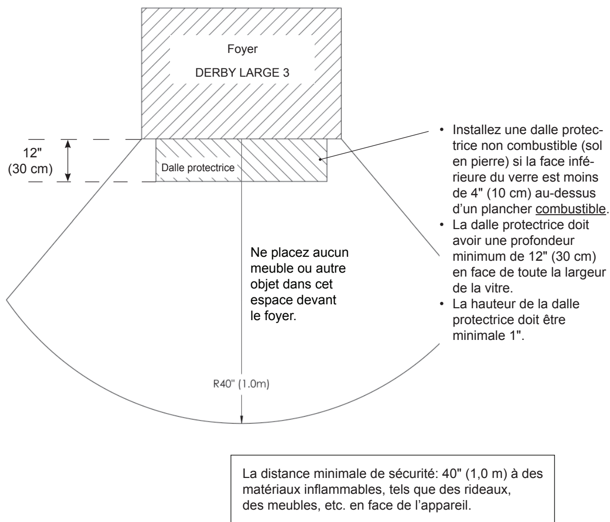
Figure 8: Distance de sécurité devant l'appareil
