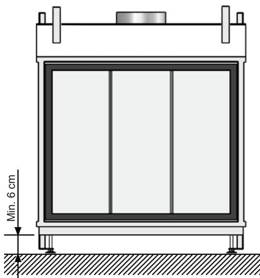
Figure 15: 6 cm au minimum entre le sol et l'appareil en bas
