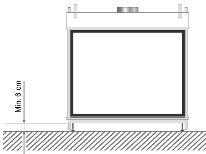
Figura 15: Mínimo 6 cm entre el suelo y la base del aparato
