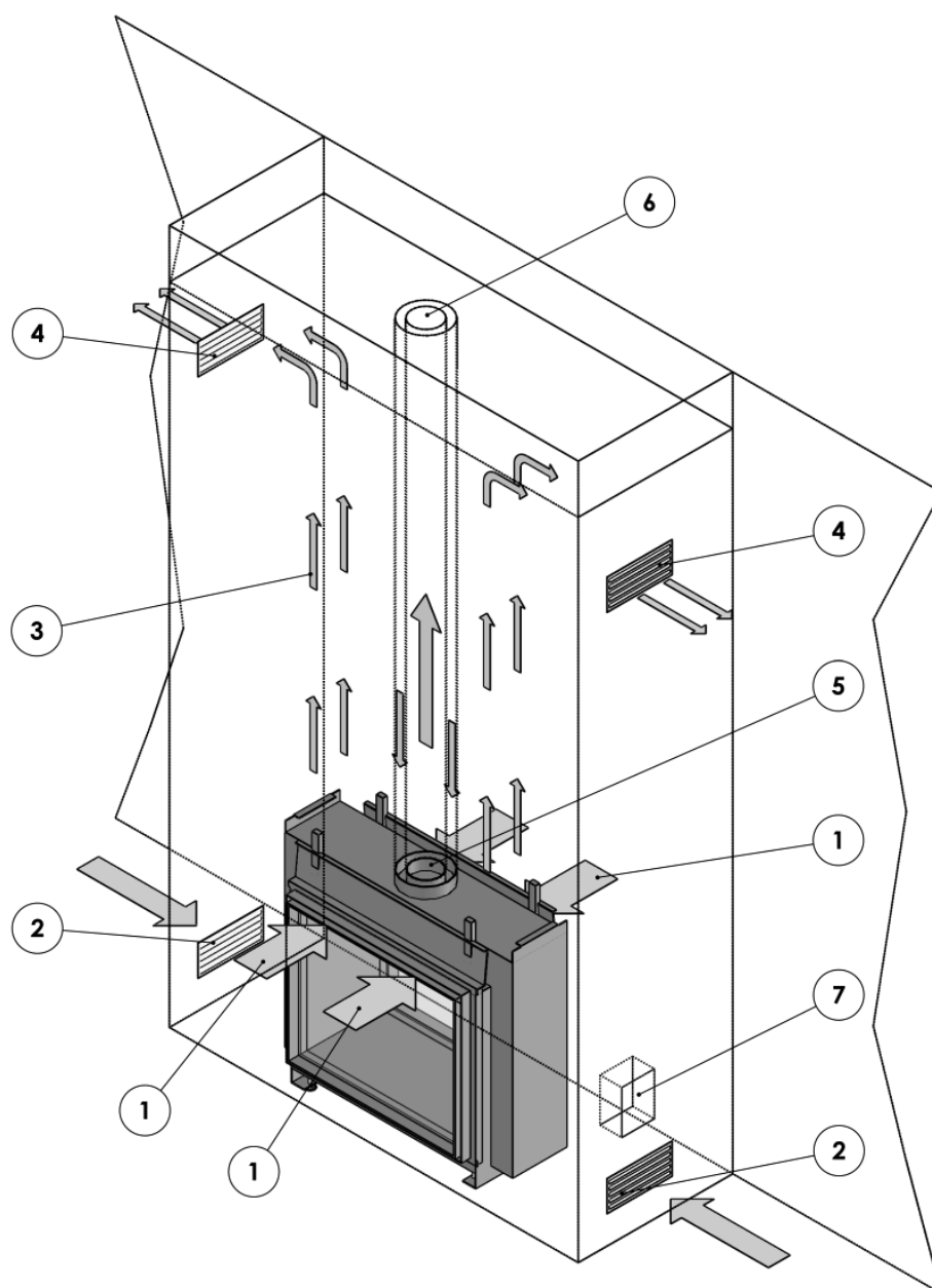
Figura 17: Aparato instalado dentro de una chimenea ventilada Salida vertical de evacuación de gases de combustión/ suministro de aire de combustión a través del techo. Aplicación sin set de convección
