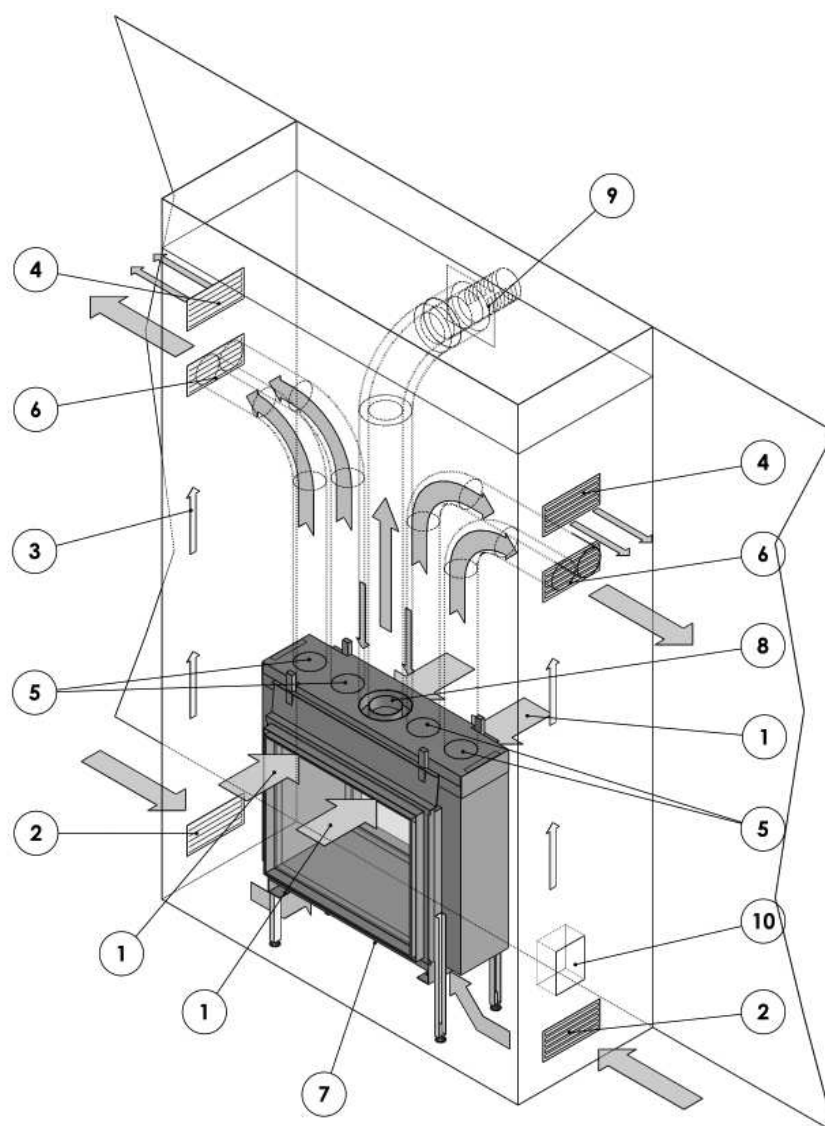
Figura 16: Aparato instalado dentro de una chimenea ventilada Salida horizontal de evacuación de gases de combustión/aire de combustión suministrado a través de la pared. Equipado con las opciones / accesorios: • Set de convección (= caja de convección y 1x juego de convección) • 1x juego de convección adicional • Pies de altura ajustable
