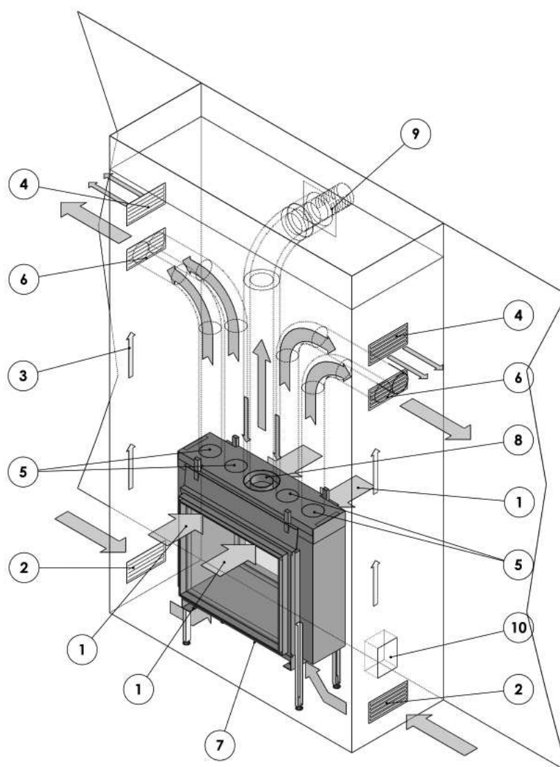
Figure 16: Appareil installé dans une cheminée ventilée Sortie horizontale de l'évacuation des gaz de combustion / l'alimentation en air de combustion par le biais du mur.
