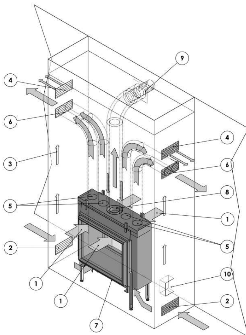
Figuur 16: Toestel ingebouwd in geventileerde schouw Horizontale uitmonding van de rookgasafvoer/verbrandingslucht- toevoer via de muur.
