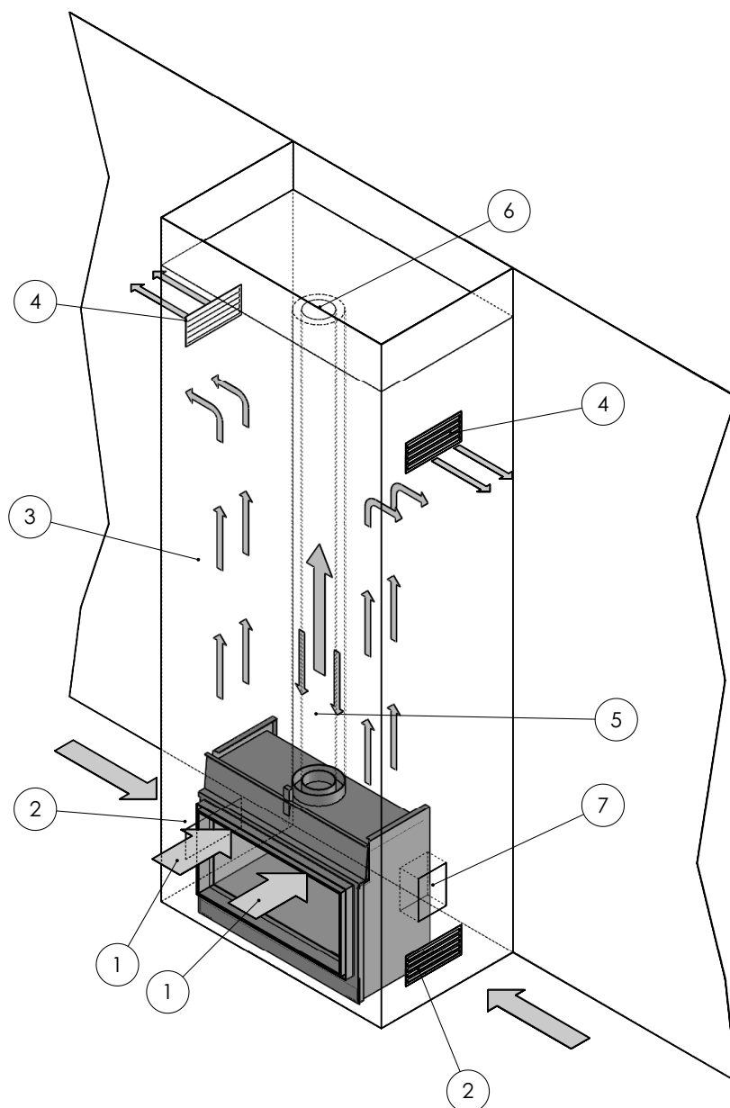
Abbildung 18: Gerät in belüfteten Kaminmantel eingebaut Vertikaler Abzug der Zu-/Abluft über das Dach. Verwendung ohne Konvektionspaket.
