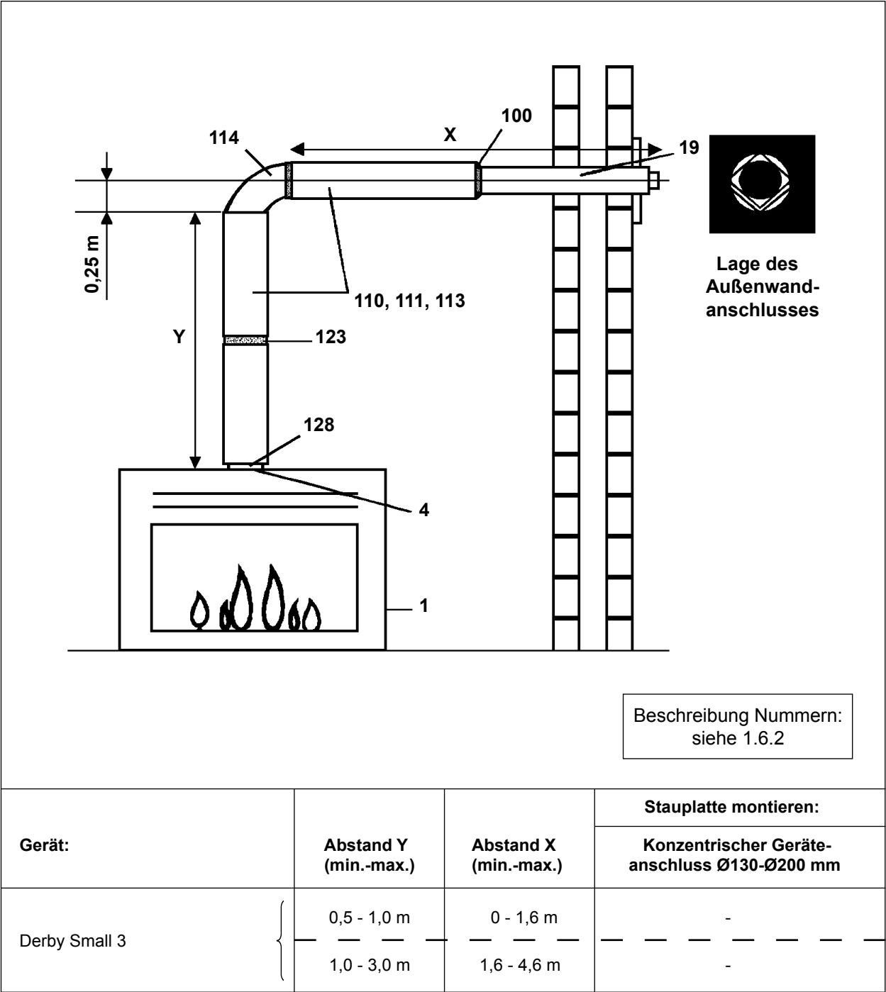
Abbildung 13: Horizontaler Außenwandanschluß
