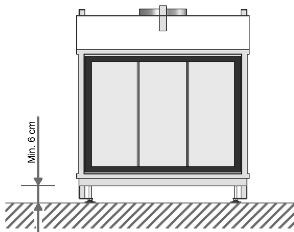
Abbildung 16: Minimal 6 cm Spiel zwischen die Unterseite des Geräts und dem Boden
