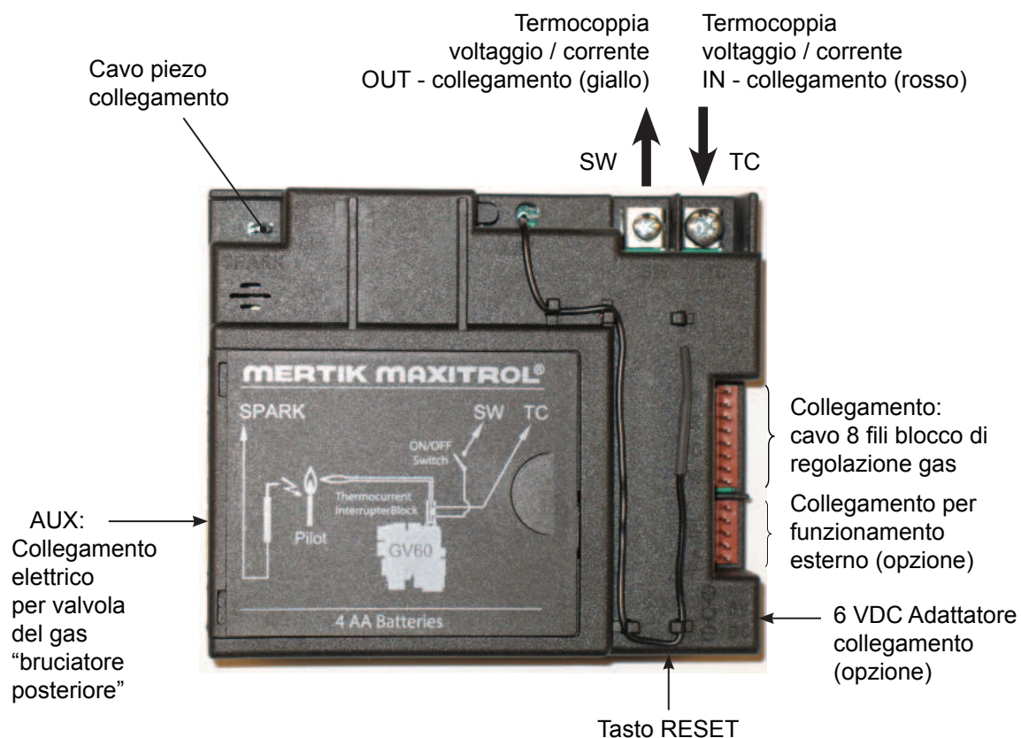
Figura 22: Ricevitore - Alto
