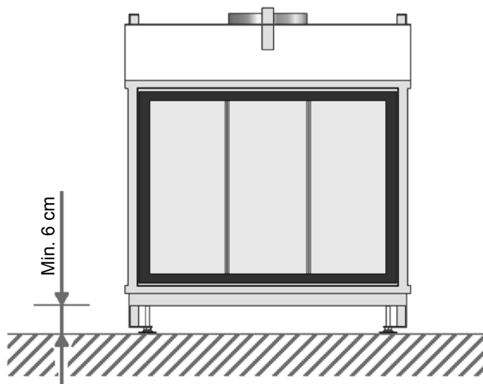
Figuur 15: Minimaal 6 cm ruimte tussen onderzijde toestel en vloer
