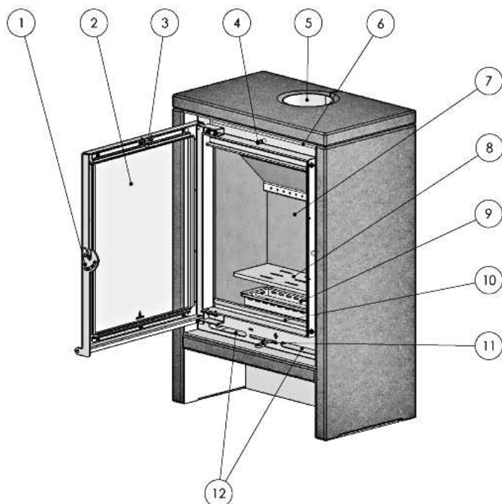
Figuur 1: Bediening
