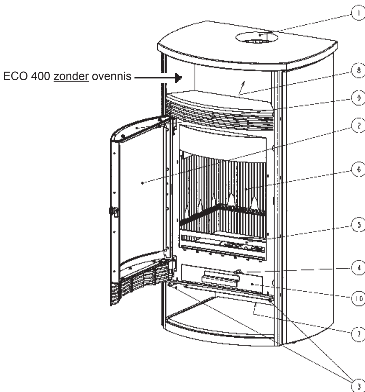
Figuur 2: Bediening
