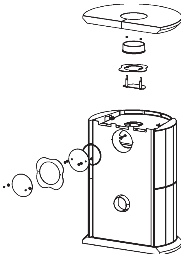
Abbildung 1: Anschluss an der Oberseite
