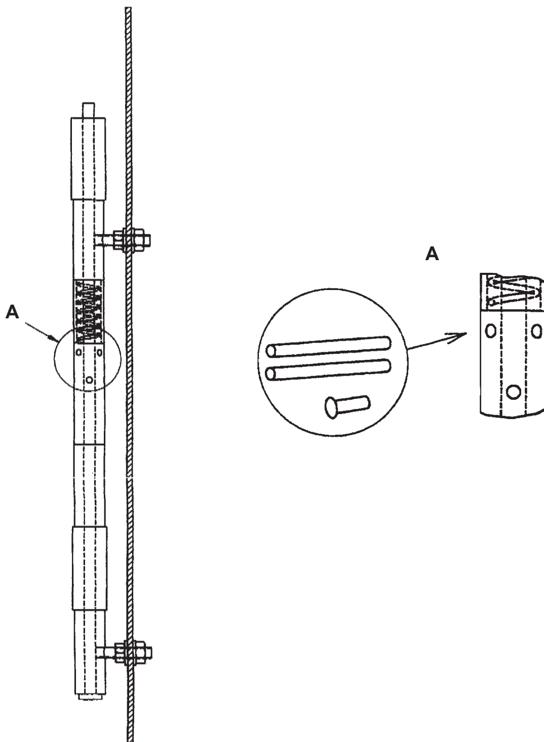
Abbildung 5: Schlüssel für Anziehen des Scharniers
