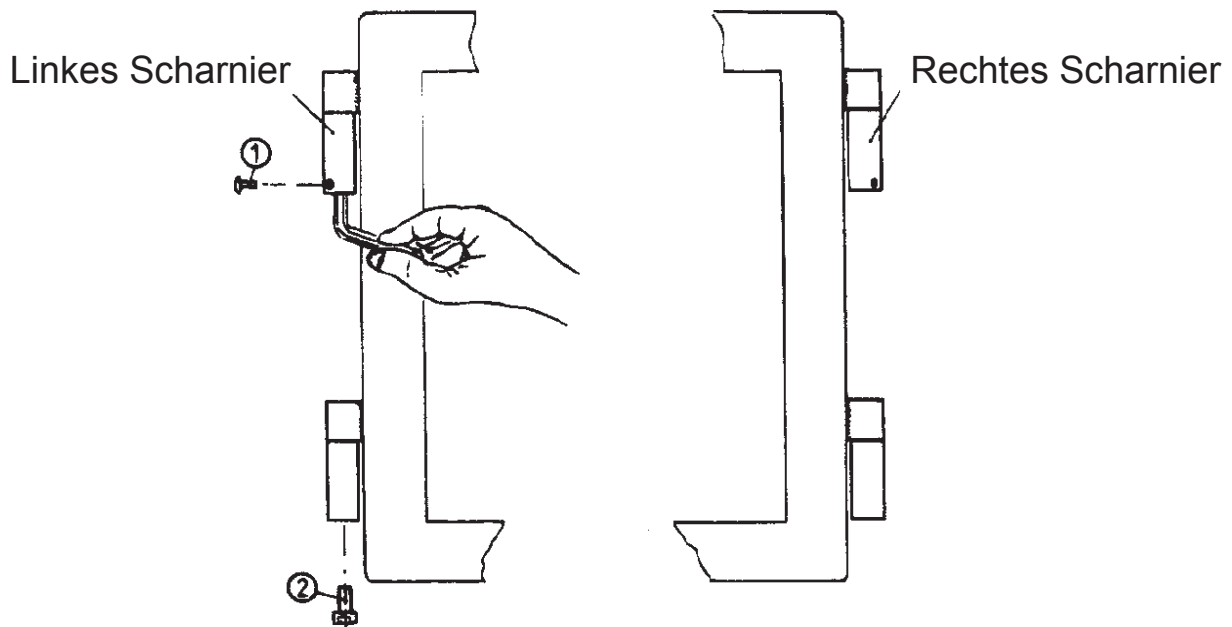
Abbildung 4: Scharnieres
