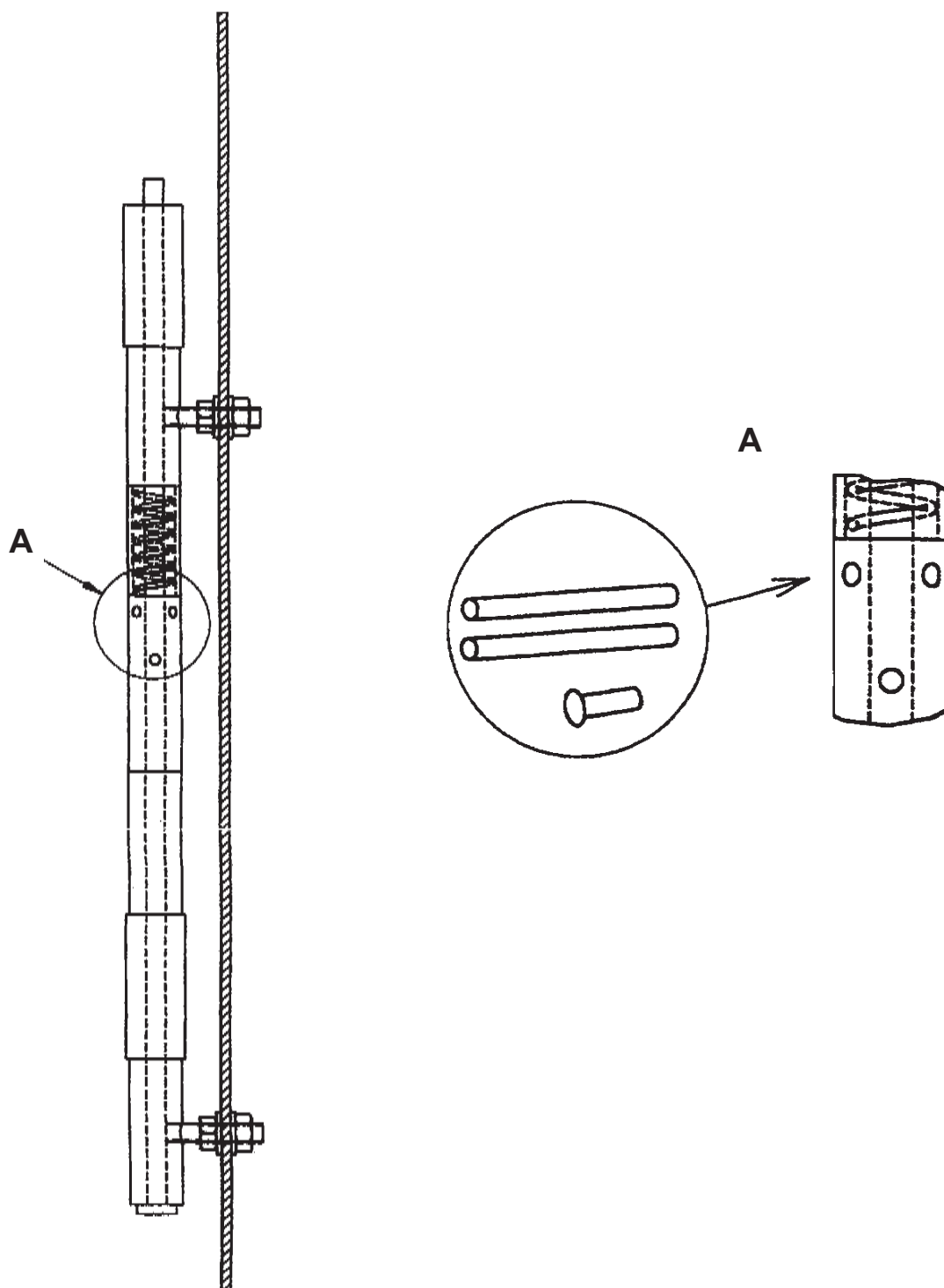
Figuur 5: Stiften in het scharnier
