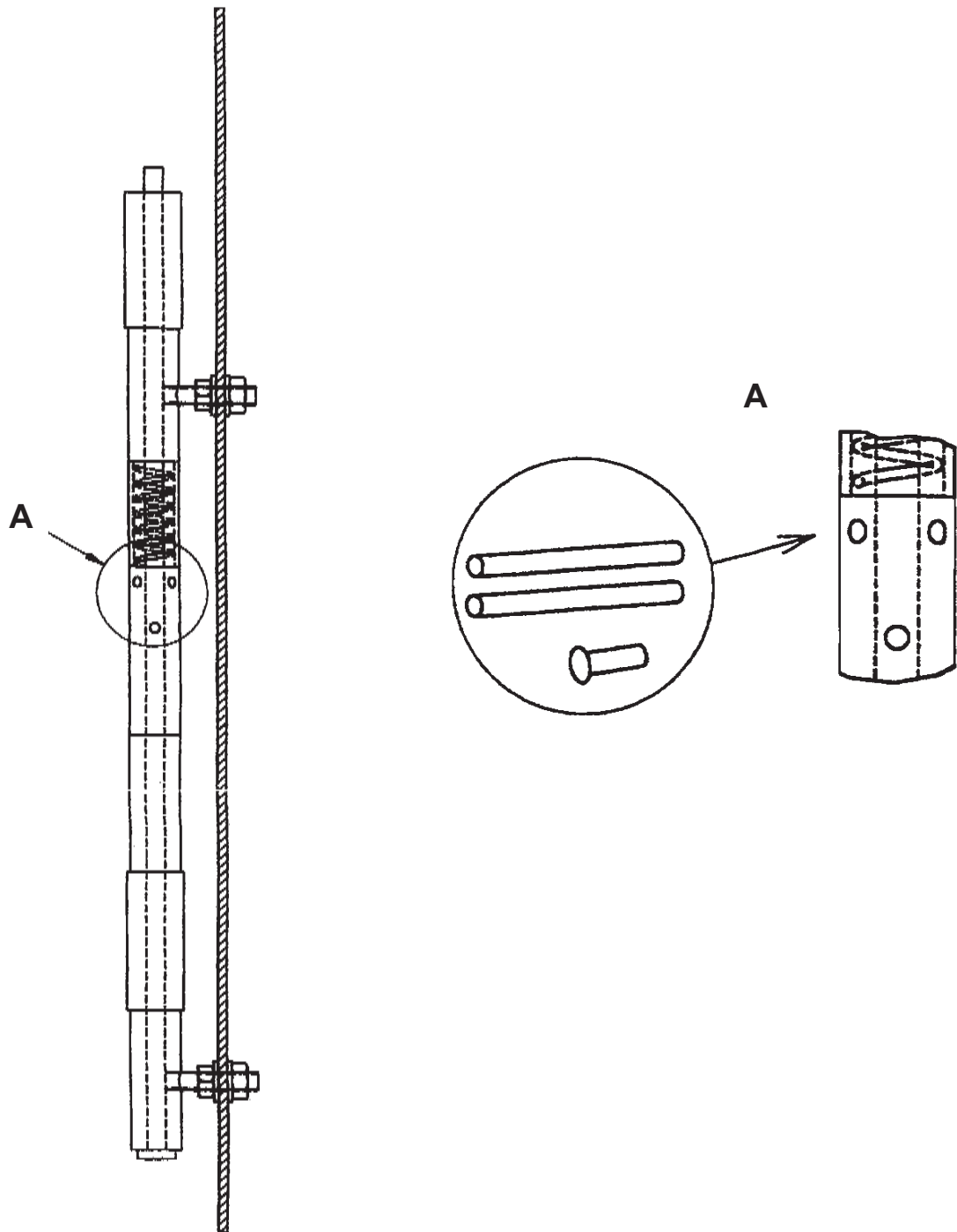
Abbildung 5: Schlüssel für Anziehen des Scharniers
