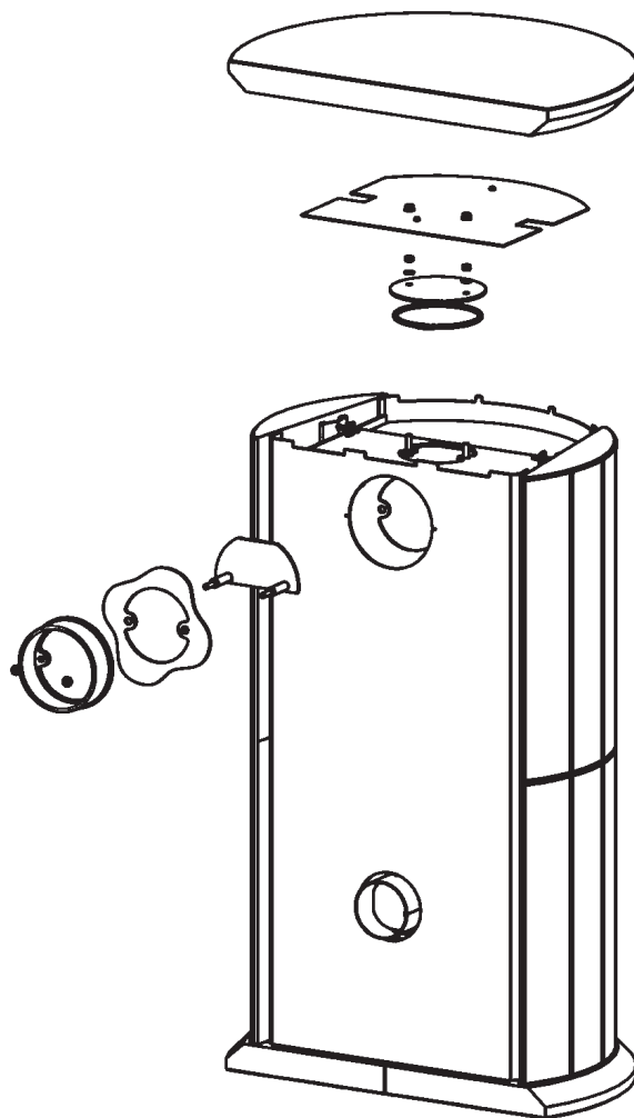
Abbildung 2: Anschluss an der Rückseite
