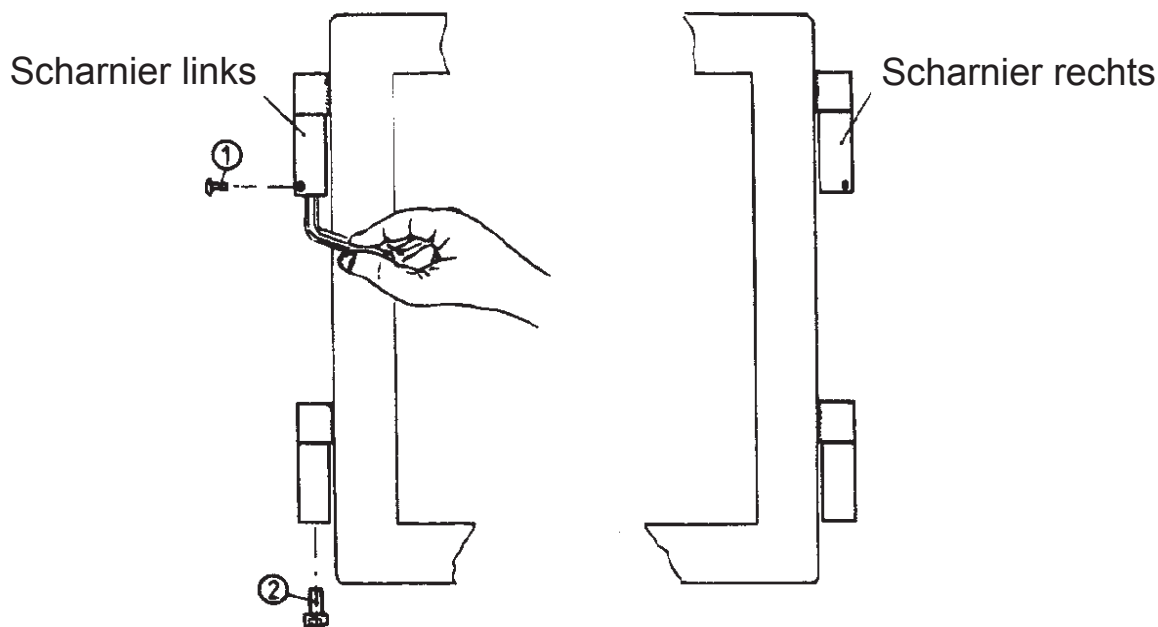
Figuur 4: Scharnieren
