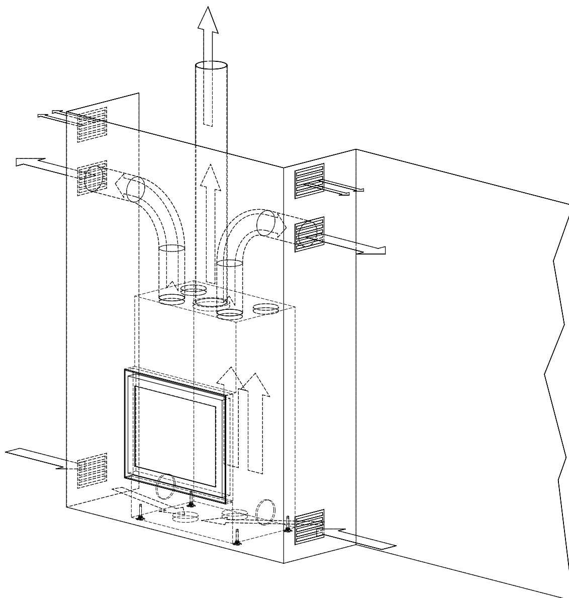
Abbildung 1: Verwendung des Konvektionssets. Be/Entlüftung und Verbrennungsluftzufuhr über den Kaminmantel.
