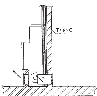
Chimenea contra un muro no inflamable y que actúa como soporte
