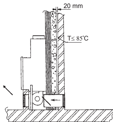
Chimenea contra un muro que actúa como soporte o contra una pared de material de construcción inflamable
