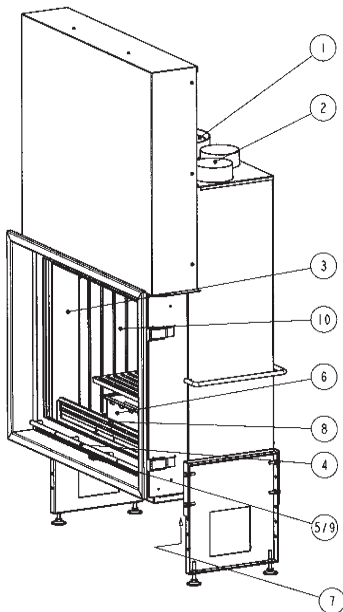
Abbildung 1: Bedienung
