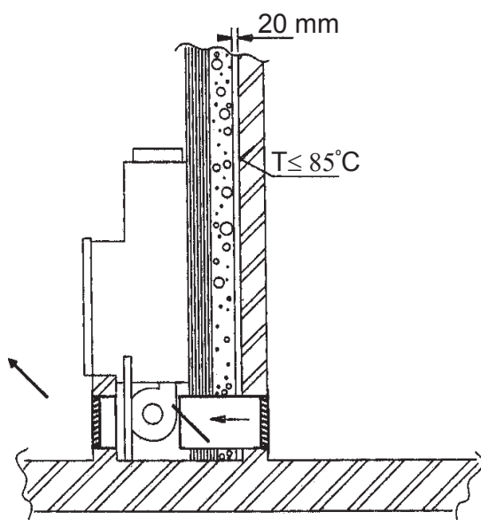
Foyer contre un mur porteur ou contre une paroi en matériaux inflammables
