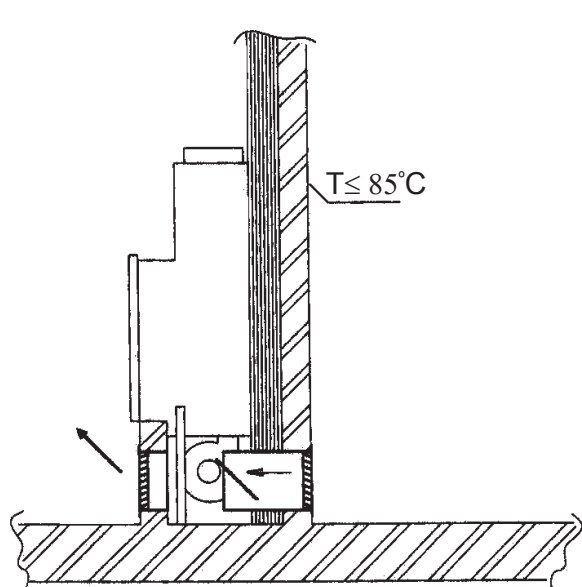
Foyer contre une paroi non porteuse et ininflammable
