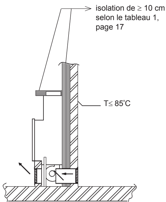
Foyer contre une paroi non porteuse et ininflammable
