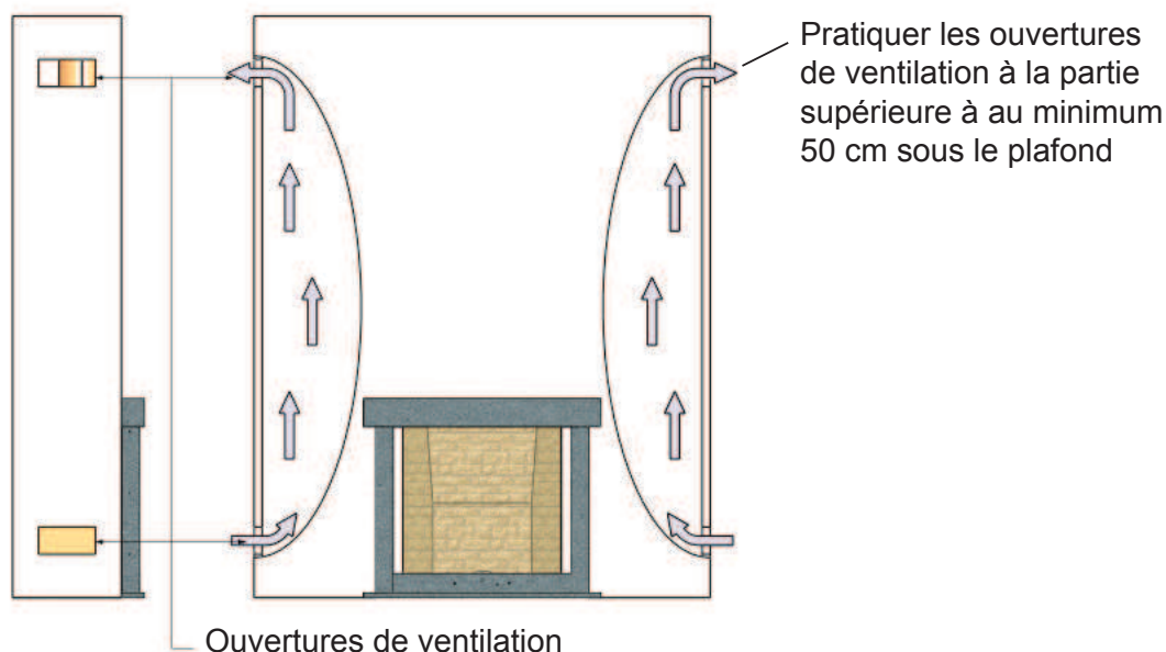
Figure 2: Application du ventilation de la cheminée
