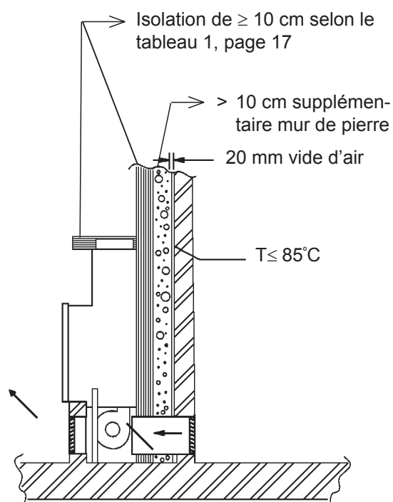
Foyer contre un mur porteur ou contre une paroi en matériaux inflammables
