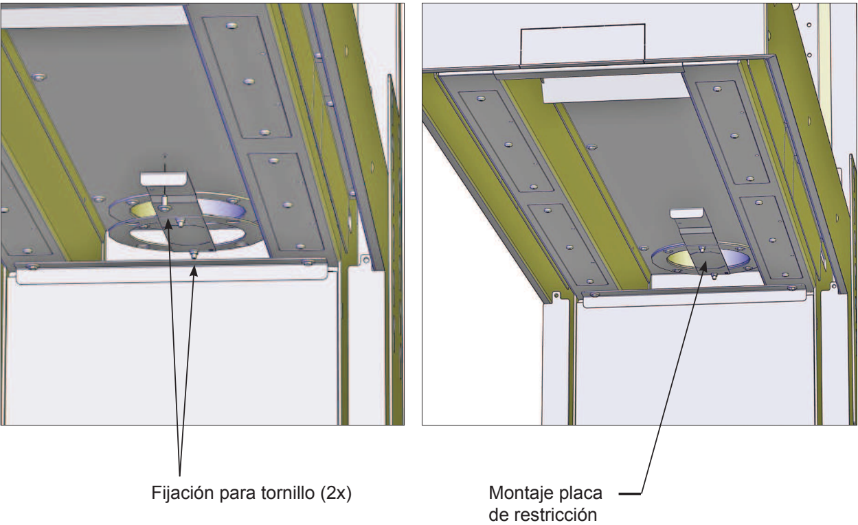
Figura 32: Colocación de la placa de restricción
