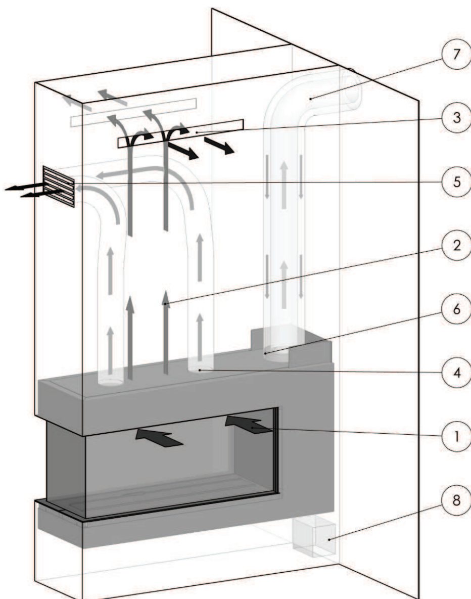
Figura 16: Aparato instalado dentro de una chimenea ventilada Salida horizontal de evacuación de gases de combustión / aire de combustión suministrado a través de la pared. Equipado con las opciones / accesorios: • Set de convección (= caja de convección y 1x juego de convección) • 1x juego de convección adicional
