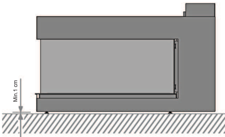
Figura 15: Mínimo 1 cm entre el suelo y la base del aparato
