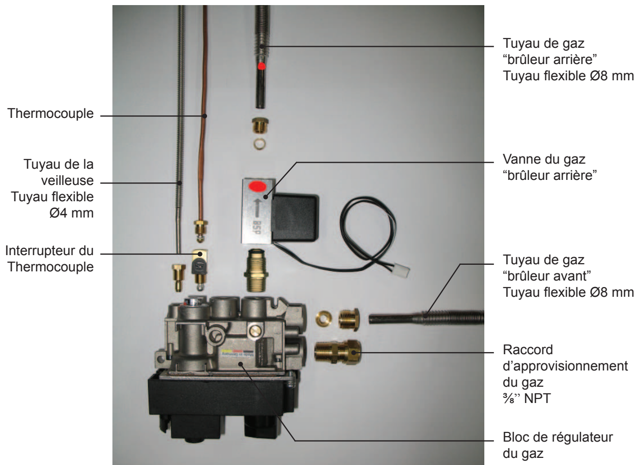
Figure 24: Bloc de régulateur de gaz et vanne de gaz: Raccords du gaz et du thermocouple
