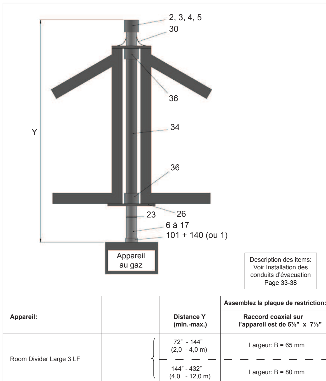
Figure 17: Terminaison verticale utilisant une cheminée munie d'une doublure existante (Flexible 4" et/ou rigide 4" x 6 5 / 8 " )
