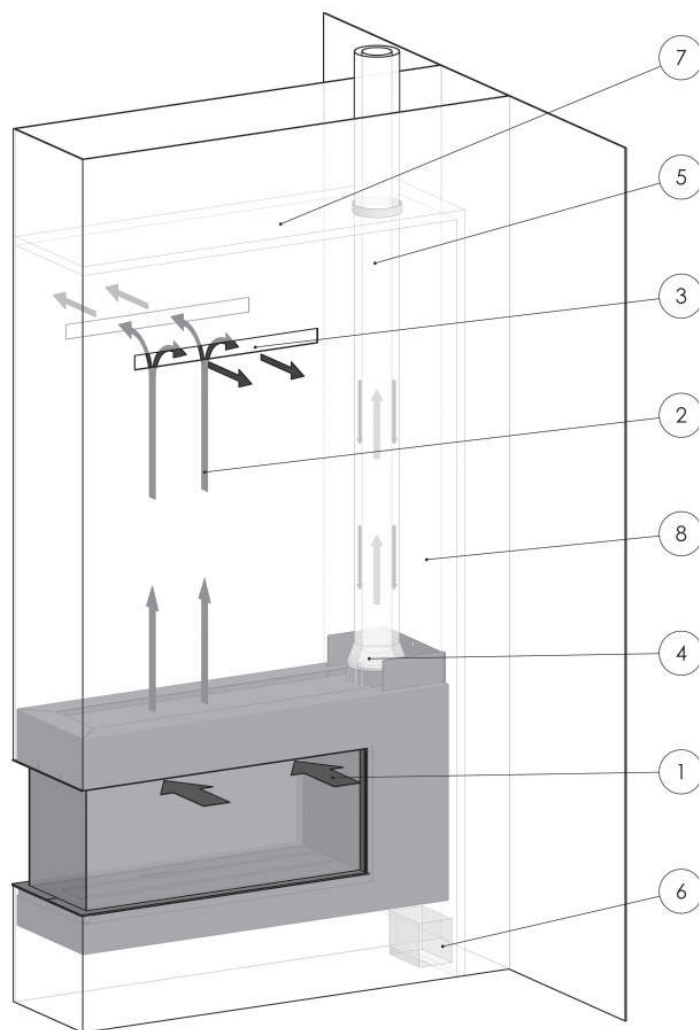
Figure 22: Appareil installé dans le manteau d'une cheminée ventilée/Enchassement Terminaison verticale d'évacuation de la fumée / source d'air de combustion au travers du toit.
