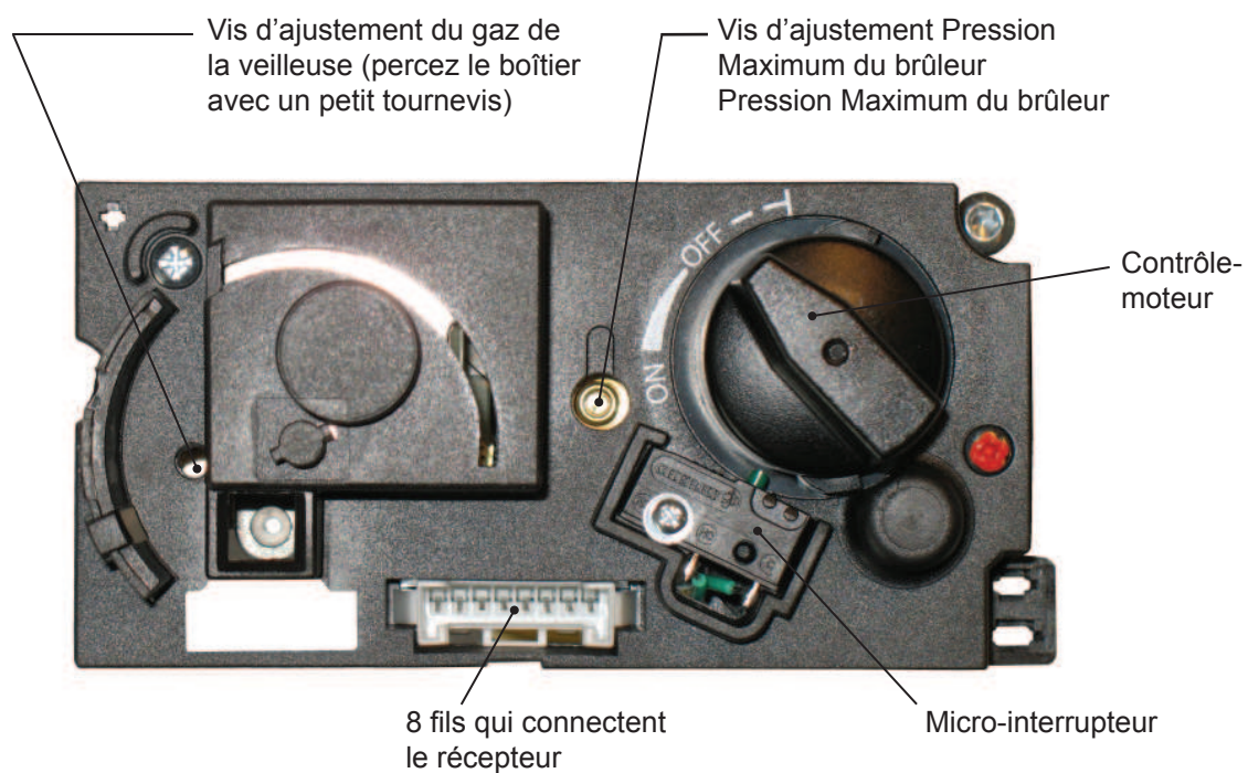
Figure 25: Bloc de régulateur du gaz - Avant
