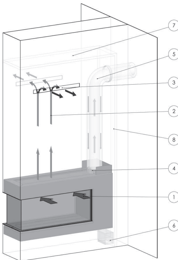
Figure 21: Appareil installé dans le manteau d'une cheminée ventilé/Enchassement Terminaison horizontale d'évacuation de la fumée/source d'air de combustion au travers du mur.
