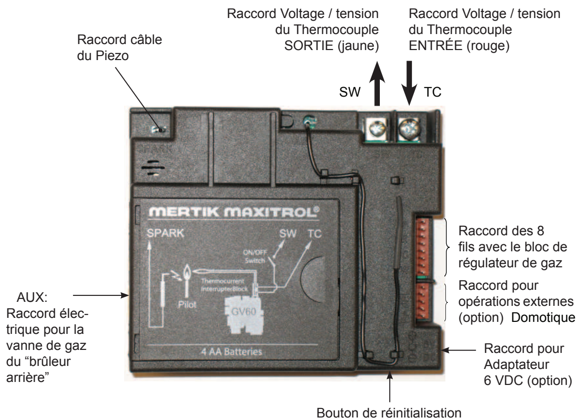
Figure 27: Récepteur - vue du dessus
