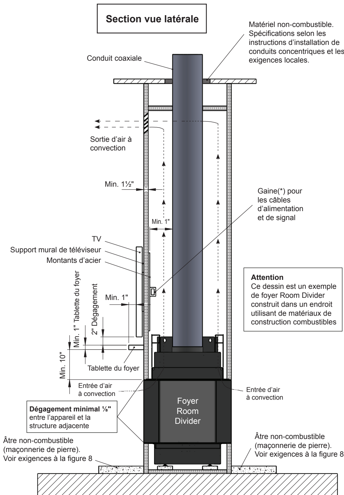
Figure 13: Installation du téléviseur au-dessus de la tablette de cheminée (Foyer plat Room Divider) (Installation en surface) - Section - vue latérale
