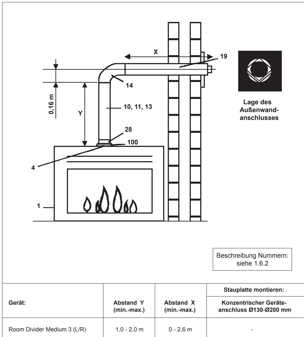
Abbildung 11: Horizontaler Außenwandanschluß
