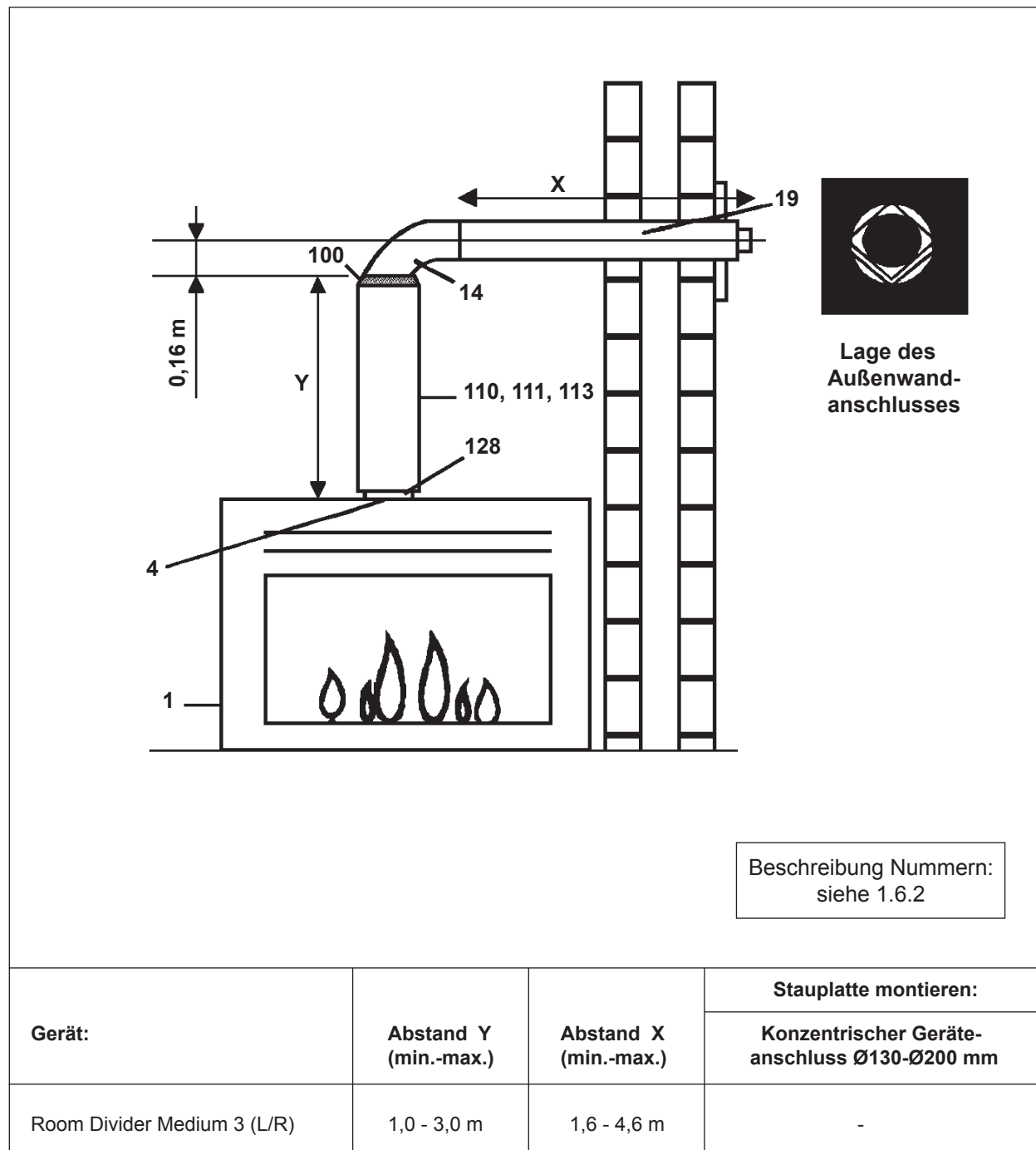
Abbildung 12: Horizontaler Außenwandanschluß
