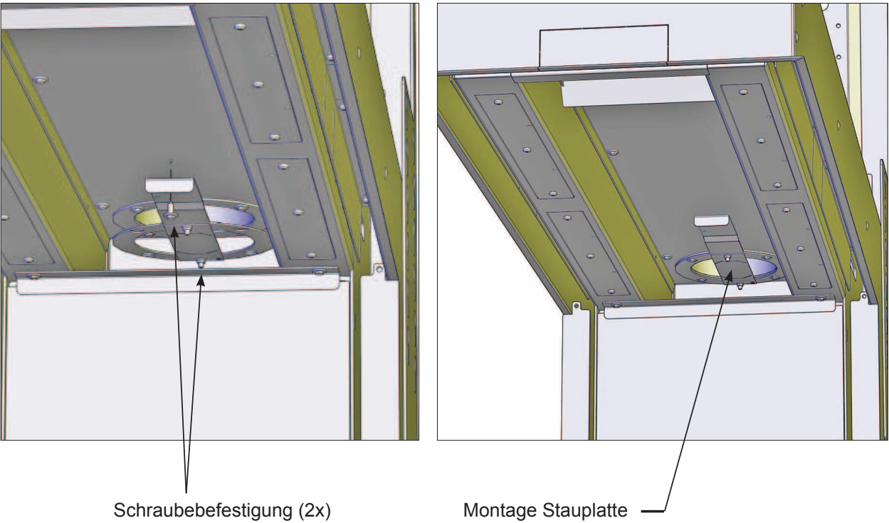
Abbildung 31: Aufstellen Stauplatte
