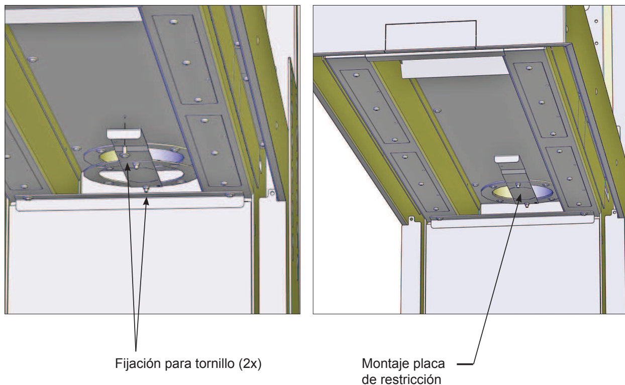
Figura 30: Colocación de la placa de restricción
