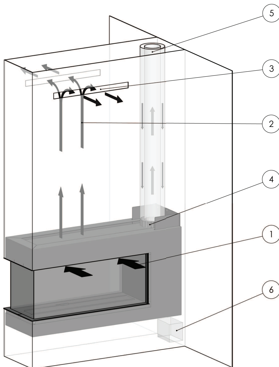
Figure 17: Appareil installé dans une cheminée ventilée Sortie verticale de l'évacuation des gaz de combustion / l'alimentation en air de combustion par le biais du toit. Application sans kit de convection.
