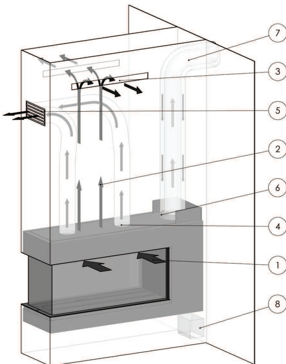
Figura 16: Apparecchio installato in canna fumaria ventilata Scarico orizzontale del gas bruciato / aria di combustione aspirata dal muro.
