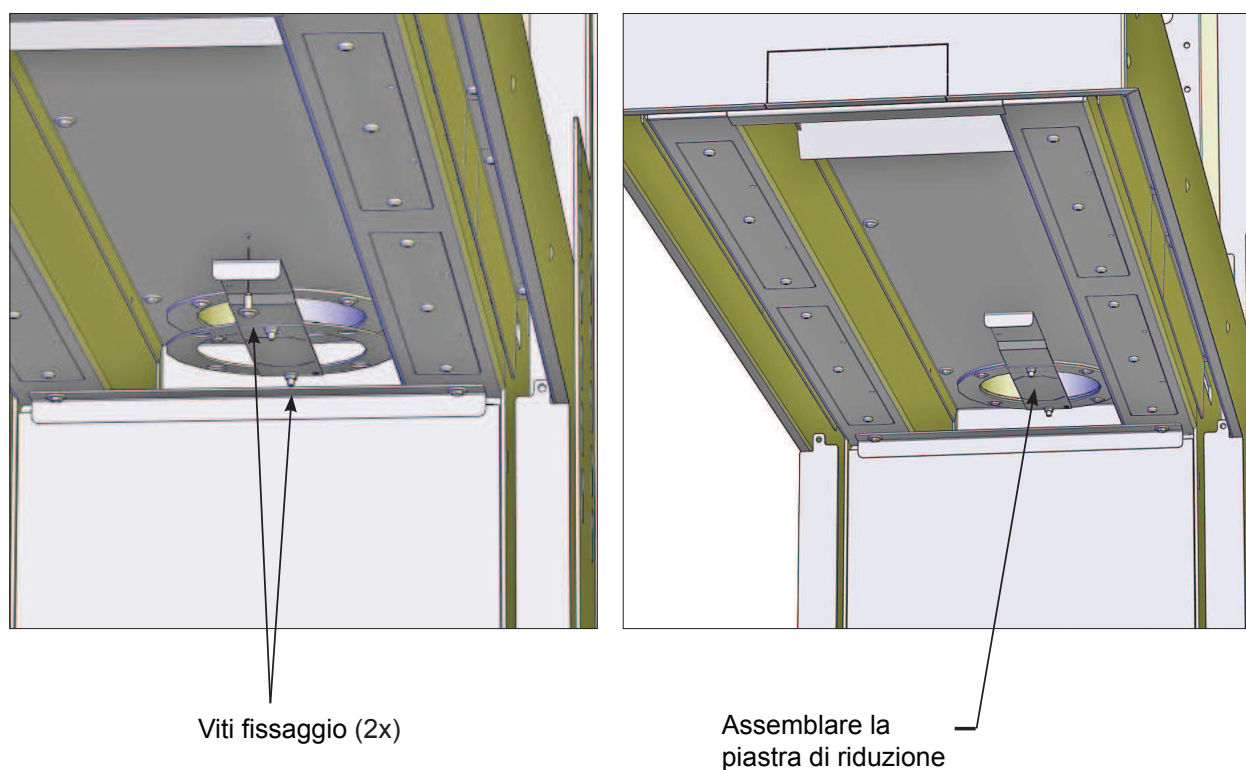
Figura 32: Assemblare la piastra di riduzione
