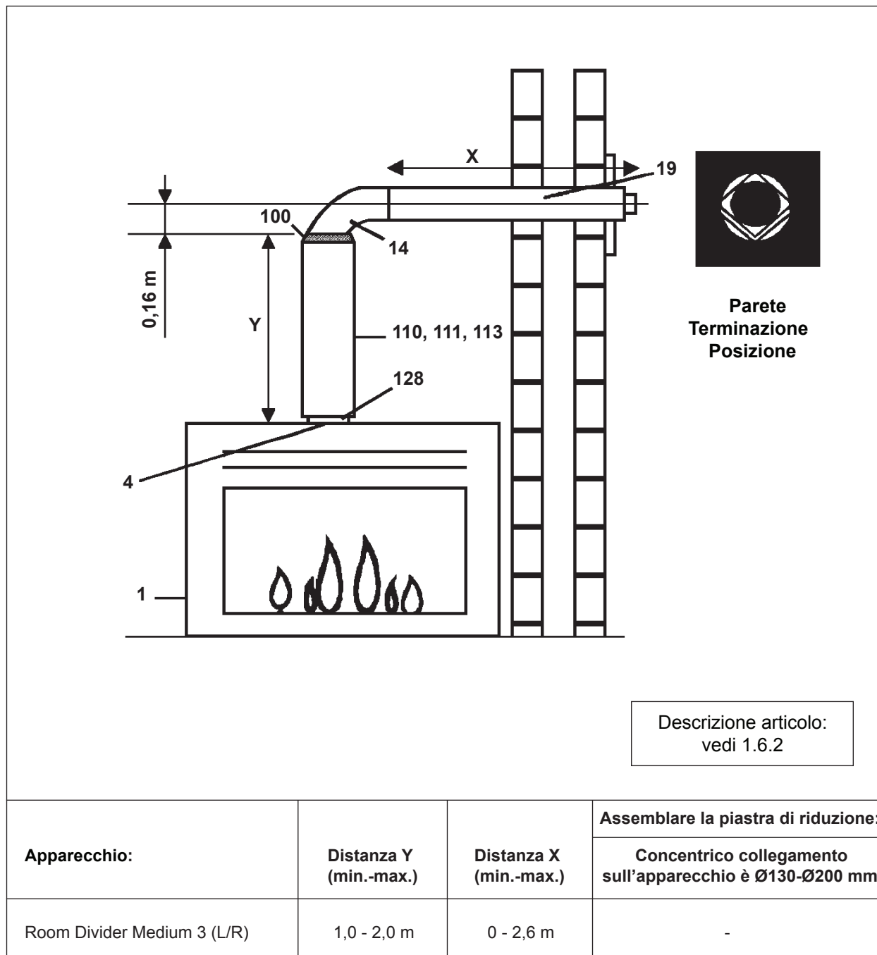
Figura 11: Terminazione muro orizzontale
