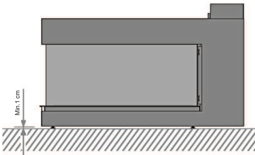
Figura 15: Deve essere mantenuto uno spazio di almeno 1 cm tra la base dell'apparecchio e il pavimento.
