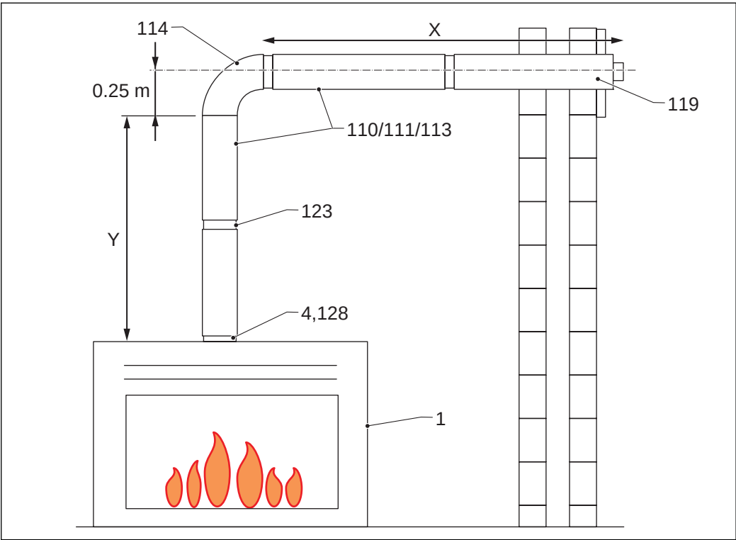
Conexión de canalización concéntrica en el aparato Ø130-Ø200 mm
