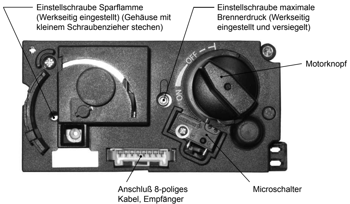
Abbildung 4: Gasregelblock
