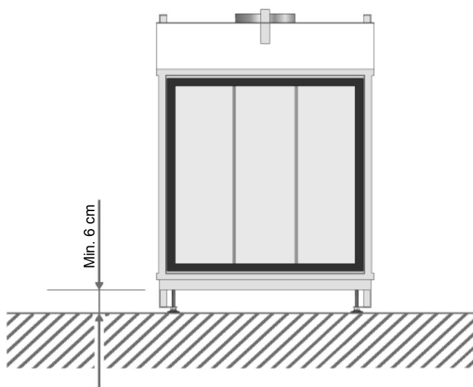
Figure 15: 6 cm au minimum entre le sol et l'appareil en bas
