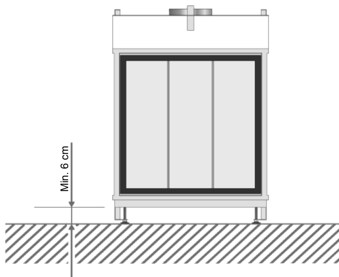
Figuur 15: Minimaal 6 cm ruimte tussen onderzijde toestel en vloer
