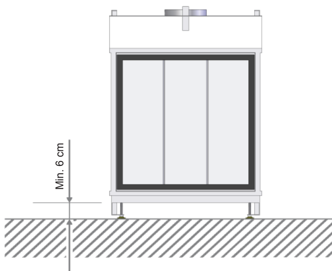
Figura 15: Deve essere mantenuto uno spazio di almeno 6 cm tra la base dell'apparecchio e il pavimento.
