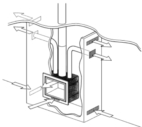
Abbildung 2: Verwendung des Konvektionssets und Be/Entlüftung des Kamins Unilux-3 55
