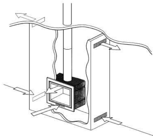
Abbildung 1: Verwendung Be/Entlüftung des Kamins Unilux-3 40
