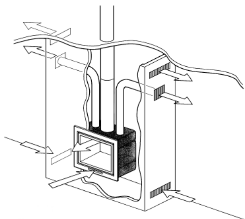
Figure 2: Application du kit de convection et ventilation de la cheminée Unilux-3 55
