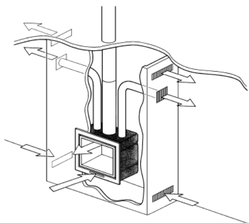
Figuur 2: Toepassing convectieset en ventilatie schouw Unilux-3 55
