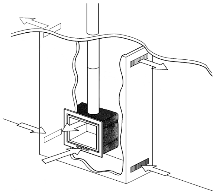
Figure 1: Application du ventilation de la cheminée
