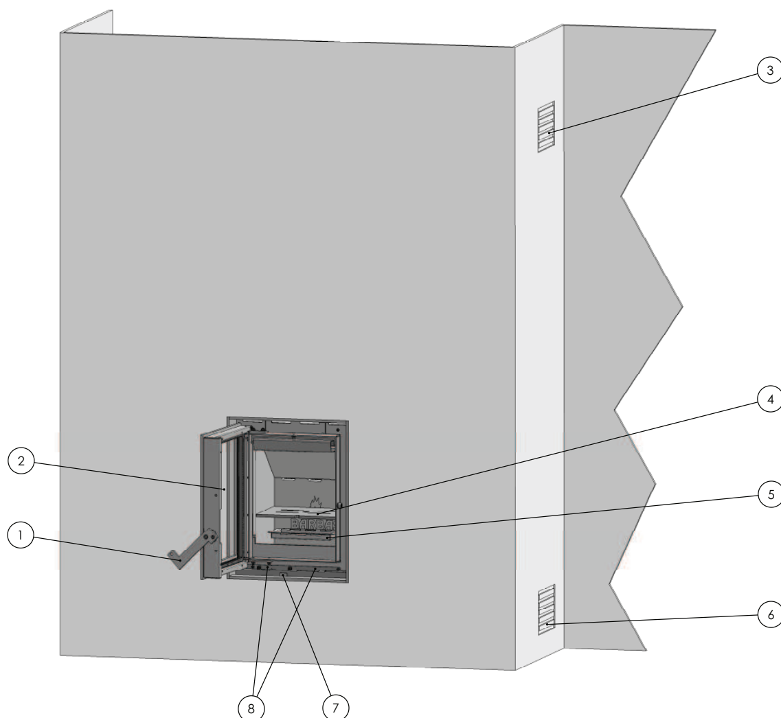
Figuur 3: Bediening
