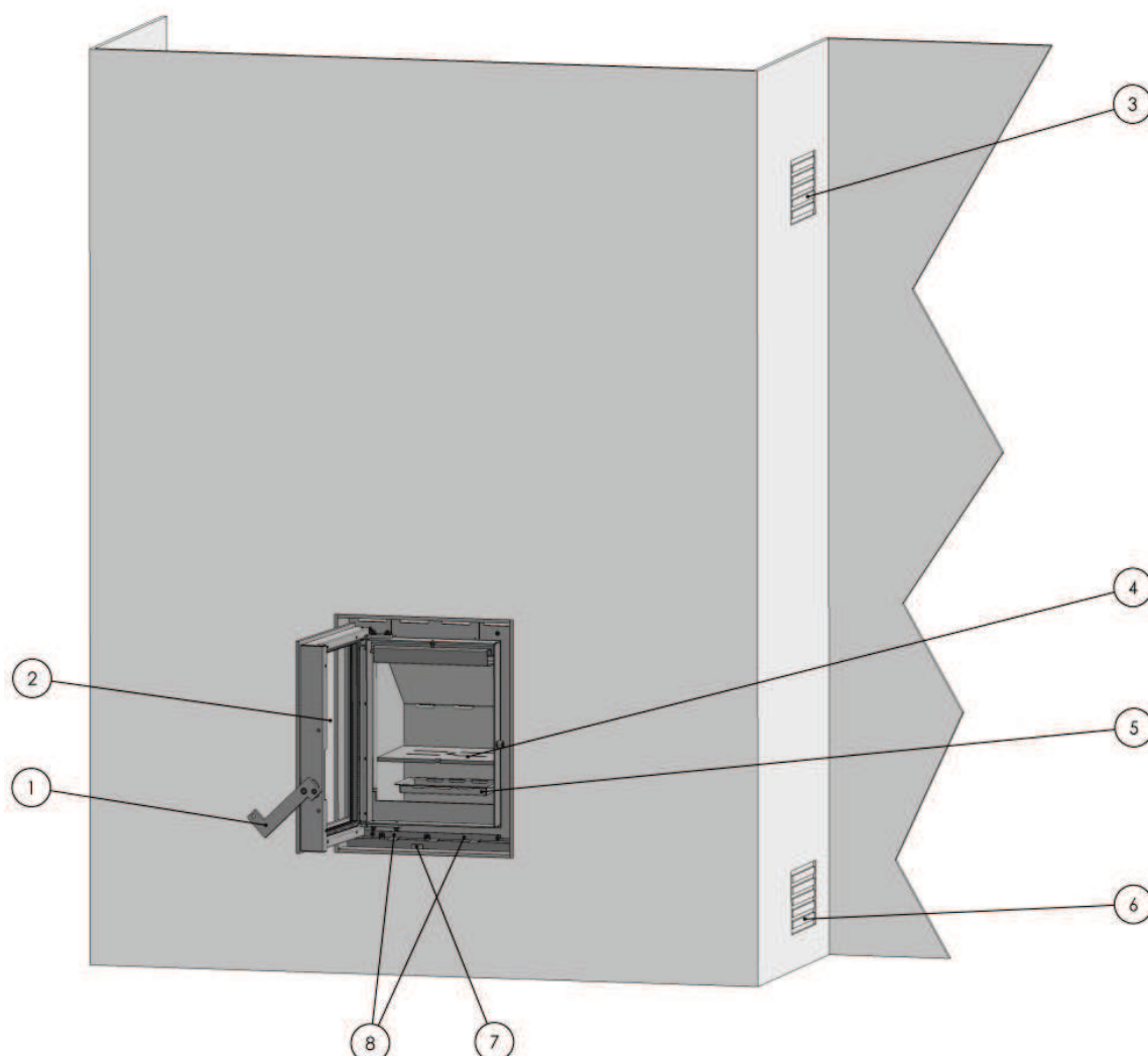
Abbildung 3: Bedienung
