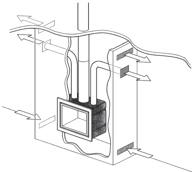
Figure 2: Application du kit de convection *) et de la ventilation de la cheminée (schématique)
