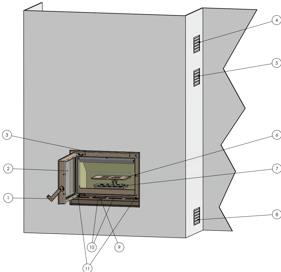
Abbildung 3: Bedienung
