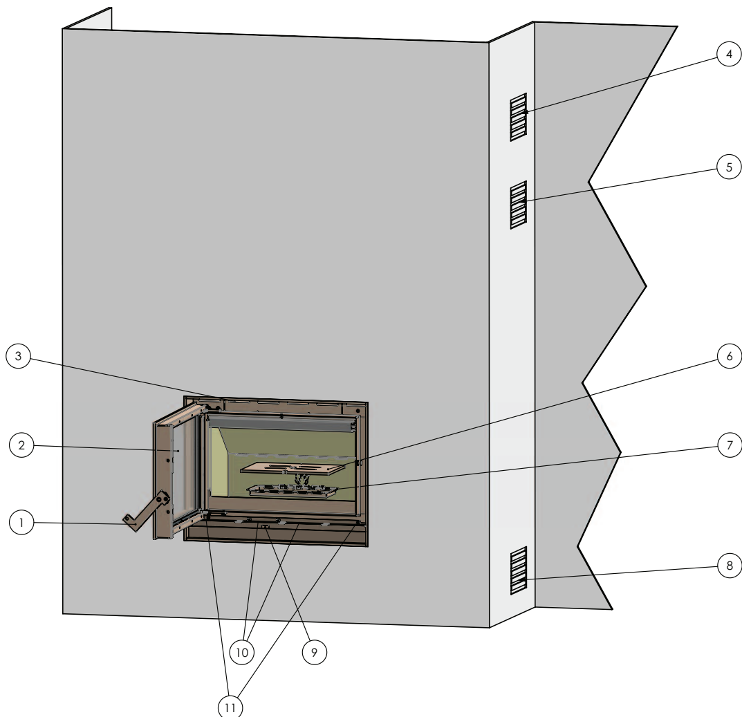
Figuur 3: Bediening
